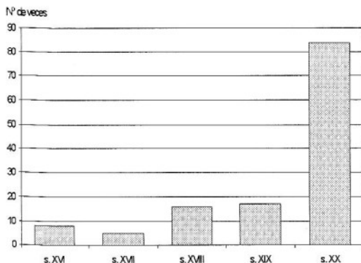
Figura 3: Número de inundaciones ocurridas en Santa Cruz de Tenerife desde 1558 hasta 2002. Fuente: Viera y Clavijo, Cioranescu, Cola, prensa escrita provincial.
