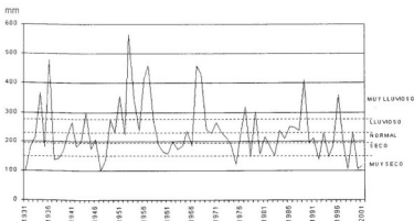
Figura 1: Calificación de la precipitación anual de Santa Cruz de Tenerife (1931-2001).
