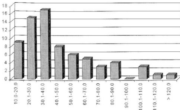
Figura 2: Frecuencia de la precipitación máxima en 24 horas en Santa Cruz (1931-2002).
