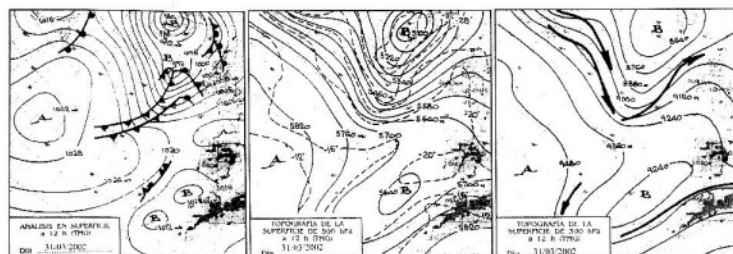
Figura 4: Mapas de superficie, 500 y 300 hPa del día 31 de marzo de 2002.
